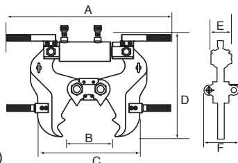
■主要寸法図
