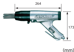
●JEX-66(日東工器) ※)コンプレッサー 5馬力以上 / 台
