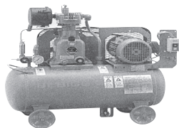
●0.75P-9.5VSA5 (日立産機システム)
