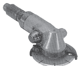
●TAG-400 (東空販売) ※) コンプレッサー 7馬力以上/台
