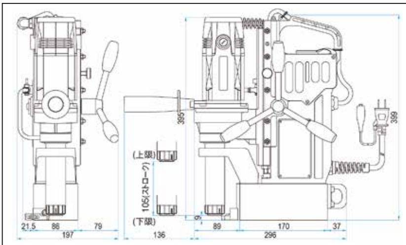
■寸法図(単位: mm)
